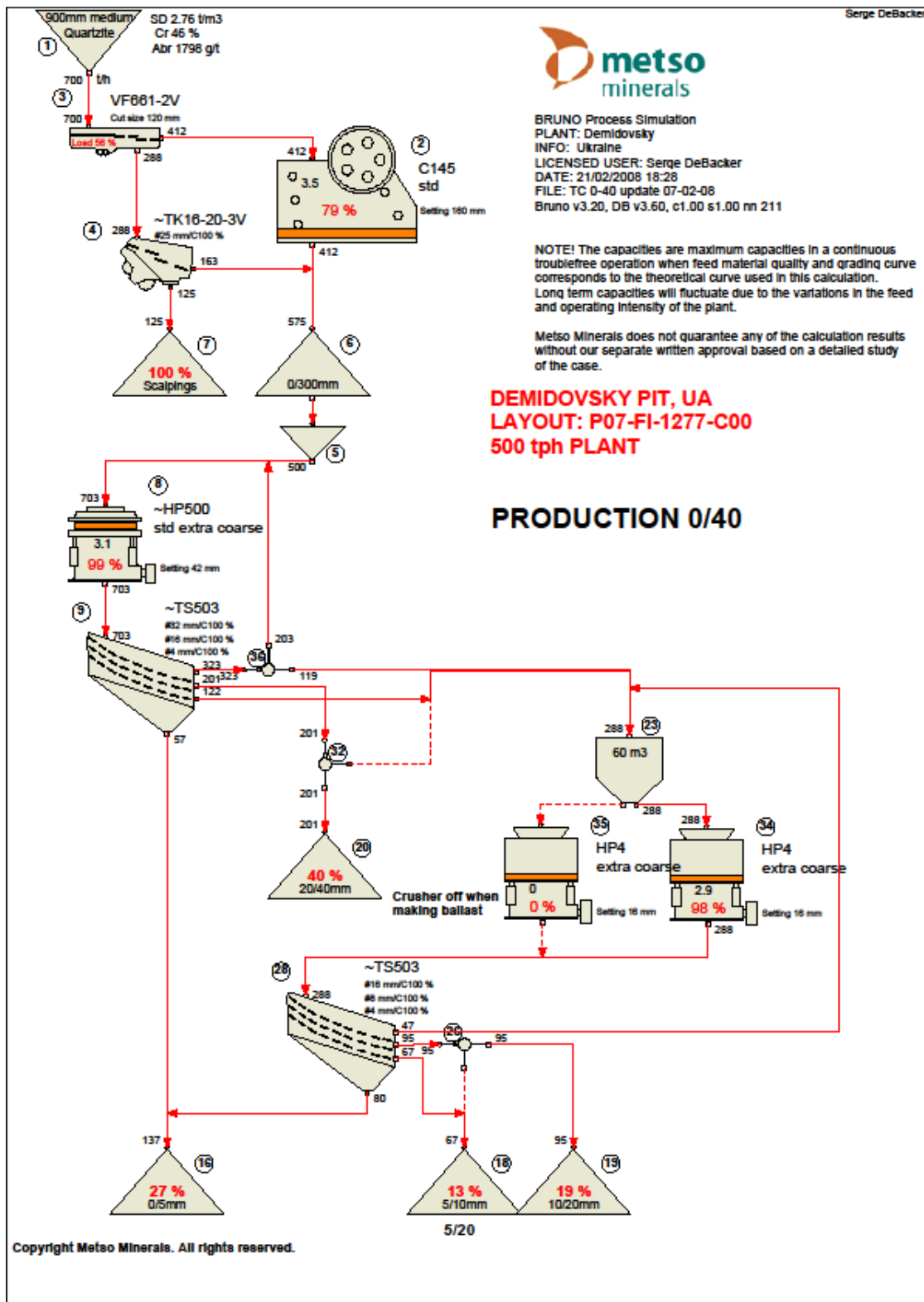
Схема технологічного процесу ДСЗ
